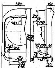
Radiateur « CITROEN » type Tracteur Dessin : 45.494
