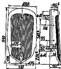
Radiateur « CITROEN » 8 CV Dessin : 45.834
