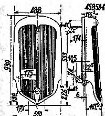
Radiateur « CITROEN » 10 CV spécial Sport Dessin : 45.850-A
