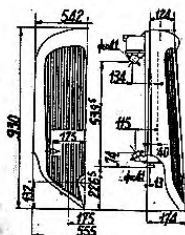
Radiateur « CITROEN » 15 CV Dessin : 45.845
