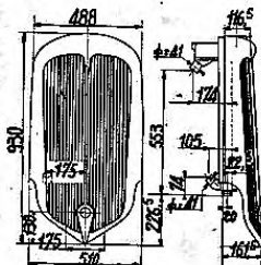
Radiateur « CITROEN » 10 CV Dessin : 45.833
