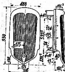
Radiateur « CITROEN » 15 CV léger Dessin : 45.840-A
