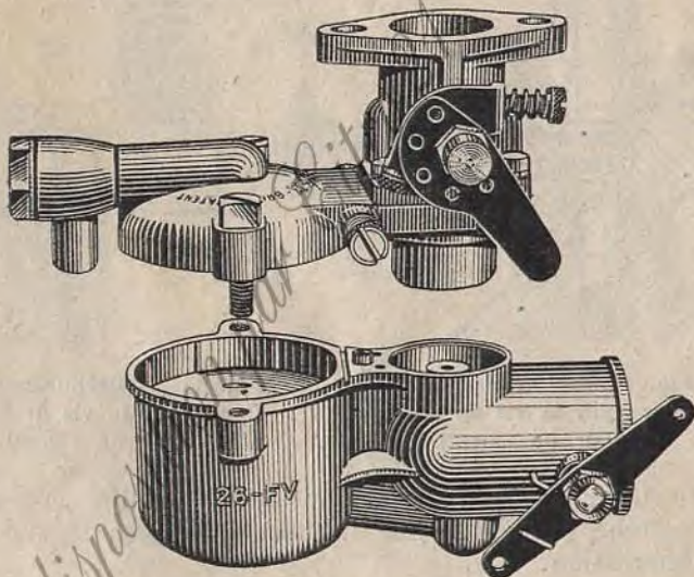
Fig. 13. — Carburateur vertical démonté.
