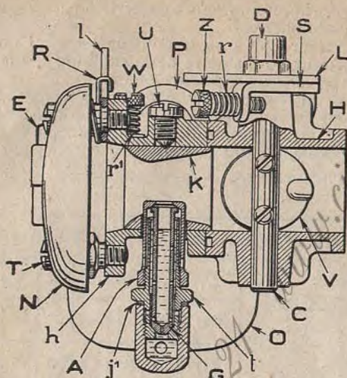
Fig. 4. — Coupe du carburateur horizontal 26 FH
