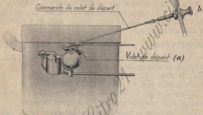
Fig. 10. — Carburateur SOLEX avec volet de départ (a) actionné par une tirette (b).
