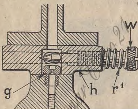
Fig. 14. — Carburateur FV. Coupe par la vis de réglage d'air du ralenti.
