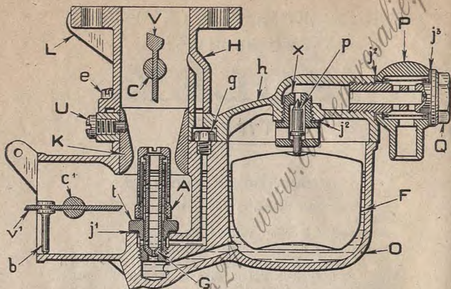
Fig 3. — Coupe du carburateur vertical Type 26 FV
