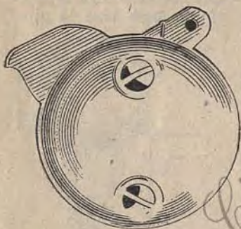
Fig. 8. — Volet de départ pour carburateurs FH horizontaux.
