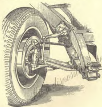
Fig. 8. — Essieu avant.
