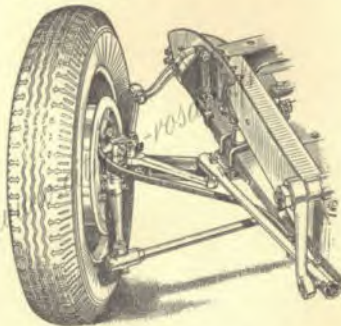
Fig. 3. — Commande de frein avant.
