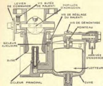
Fig. 2. — Coupe du Carburateur.
