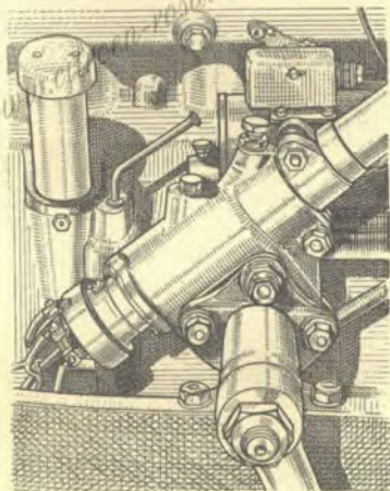
Fig. 5. — Boîtier de direction.
