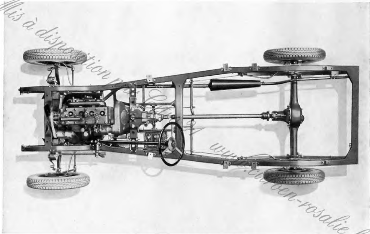
VUE EN PLAN DU CHASSIS 8 CV
