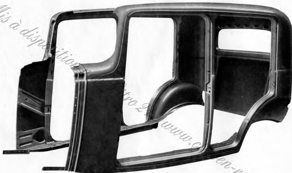
Vue des éléments assemblés.
