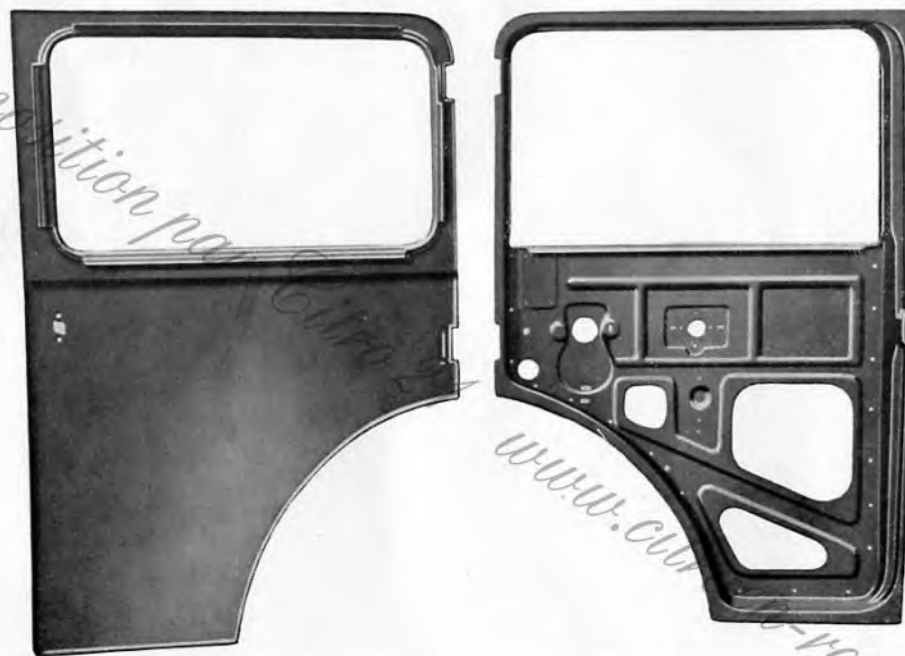
Vue d'une porte et de son panneau de renfort
