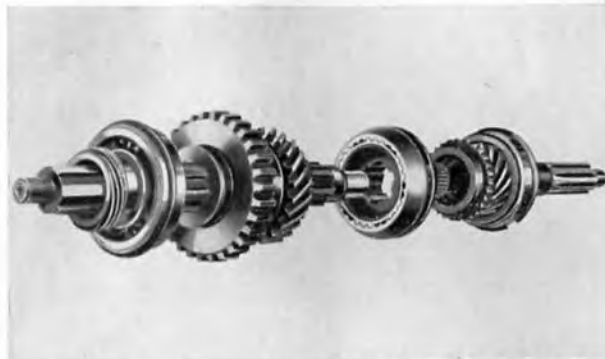
Vue des engrenages montés sur l'arbre primaire de la boîte de vitesses. A noter le synchroniseur et les clavots,
