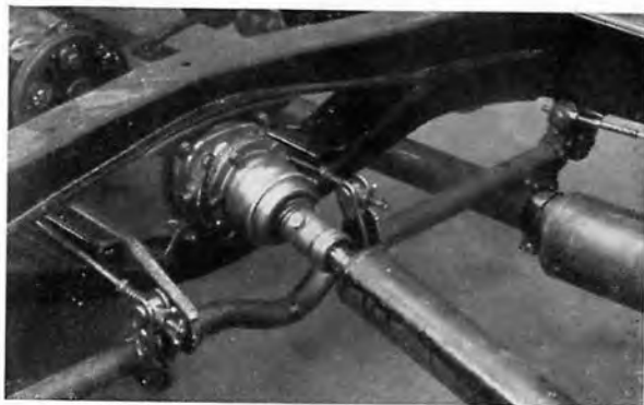
Au dessus : VUE DU RELAI DE TRANSMISSION DE LA 15 CV.
