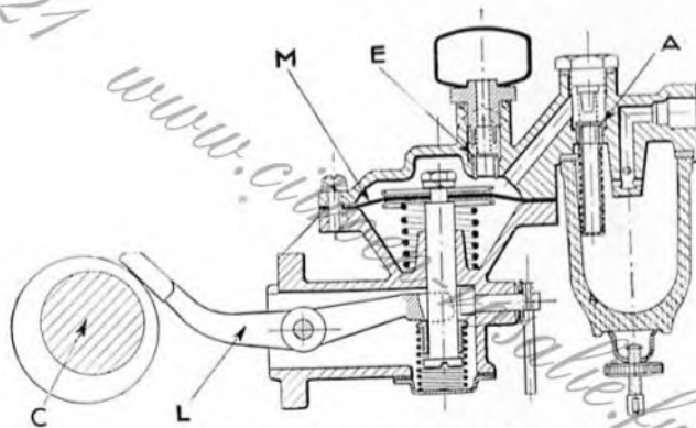
COUPE DE LA POMPE A ESSENCE
