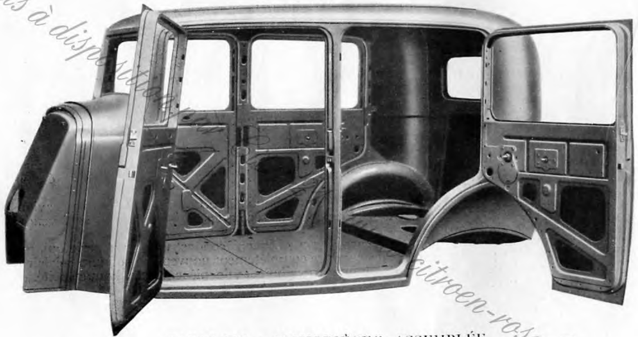
CARCASSE "MONOPIÈCE" ASSEMBLÉE
