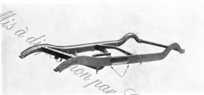
LE NOUVEAU CADRE CITROËN
