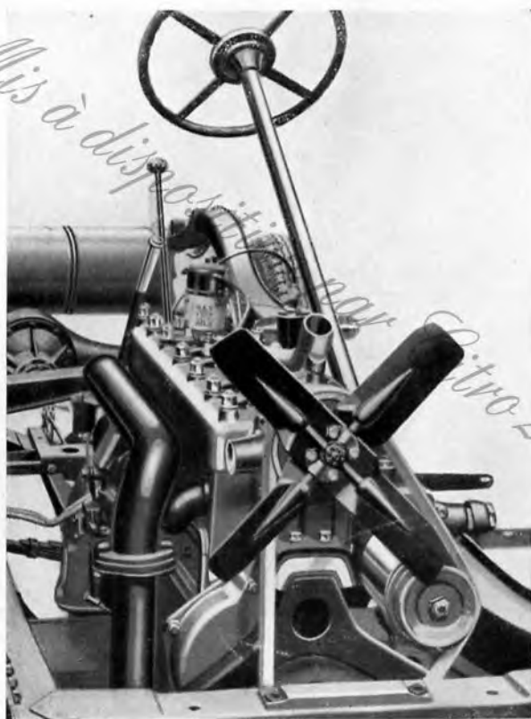
VUE DU MONTAGE "MOTEUR FLOTTANT" SUR CHASSIS 15 CV 6 CYLINDRES
