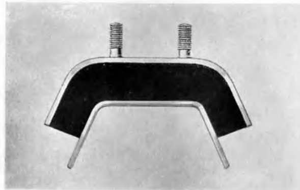
SUPPORT AVANT DU MOTEUR FLOTTANT
