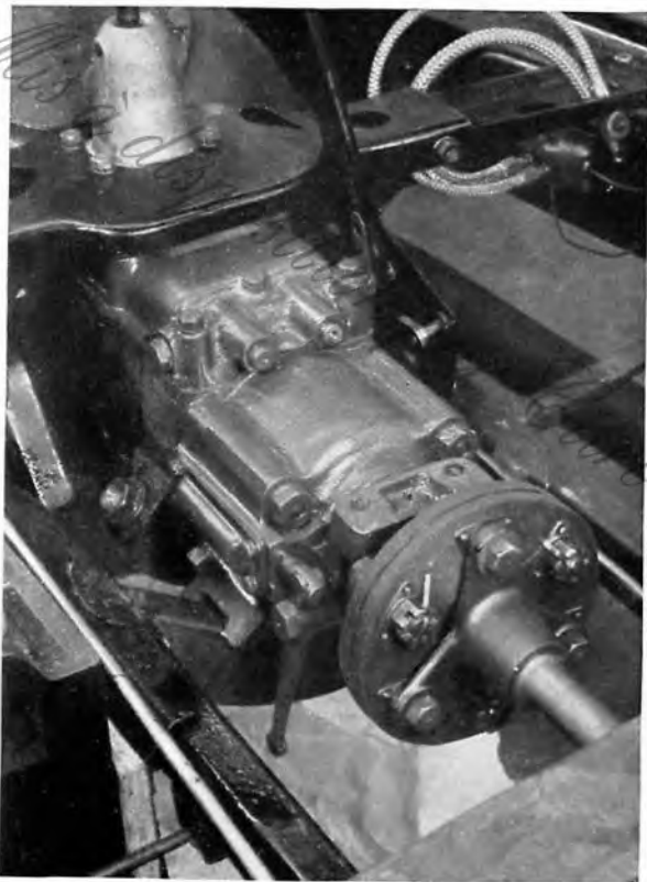
Au dessus : VUE DU RELAI DE TRANSMISSION DE LA 15 CV.
